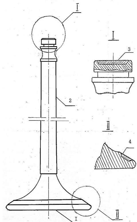
Рис. 4. Дефекты выпускных клапанов:
