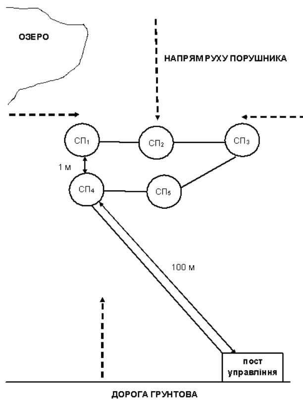
Рис. 1. Схема розміщення сейсмоприймачів для визначення дальності до людини
