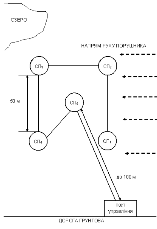
Рис. 4. Схема розміщення сейсмоприймачів для визначення напрямку і траєкторії руху порушника
