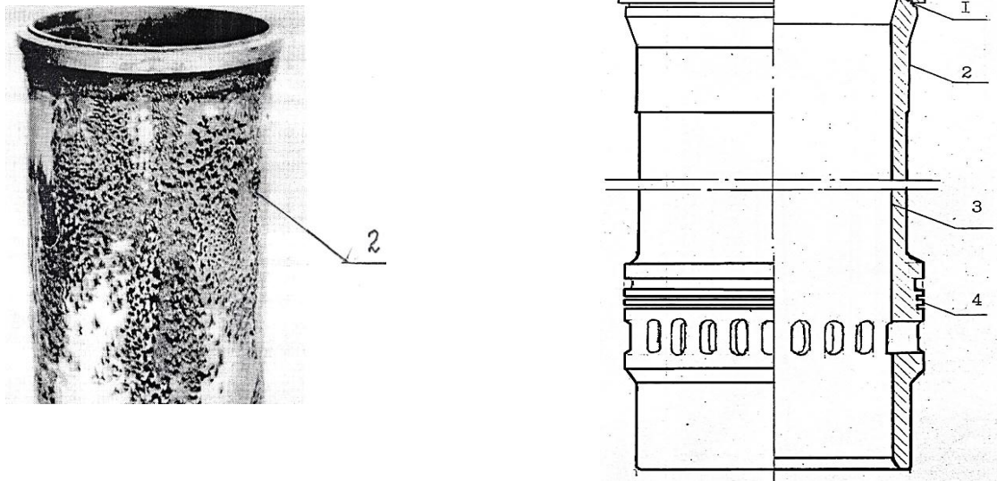
Рис. 2. Дефекты цилиндрических втулок
