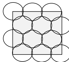
Рис. 3. Розрахунок кількості канату в 1 погонному метрі БСЗ, побудованих в 20-м глибині за принципом кольчужного плетіння
